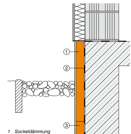
1 Sockeldämmung Polyfoam Ultragrip SE, verputzt 2 Feuchtigkeitsabdichtung 3 Perimeterdämmung
